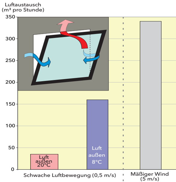
Luftaustausch an einem gekippten Fenster durch Thermik und Windeinfluss.
