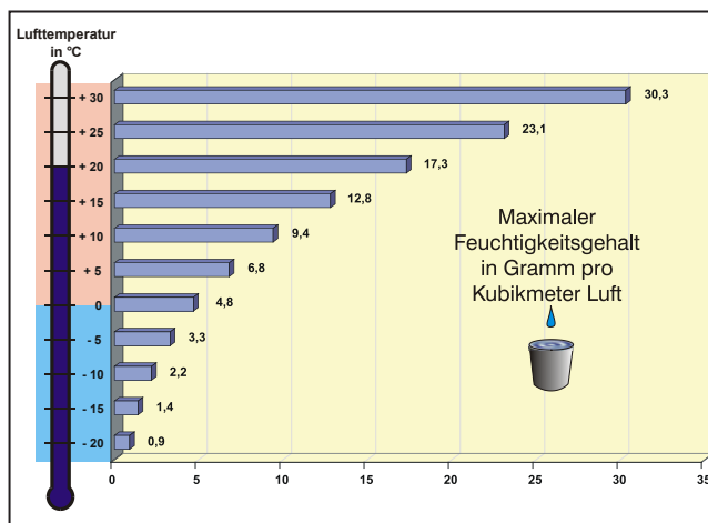
Maximaler Wasserdampfgehalt (= 100 % relative Luftfeuchte) in Gramm pro m³ Luft bei verschiedenen Temperaturen.
