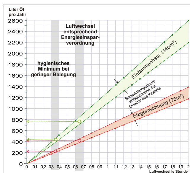
Heizenergieverbrauch für die Lüftung in Abhängigkeit von der durchschnittlichen Luftwechselrate.
