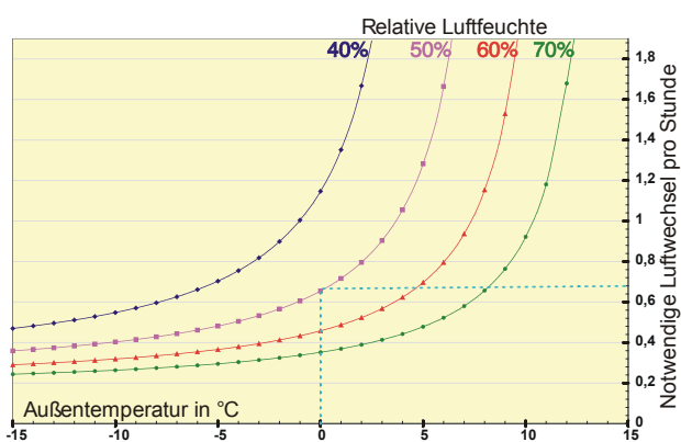
Notwendige Luftwechselraten zur Wasserdampfabfuhr in Abhängigkeit von der Außentemperatur.
