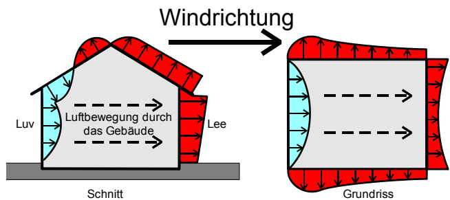
Winddruck und -sog bei einem frei stehenden Gebäude
